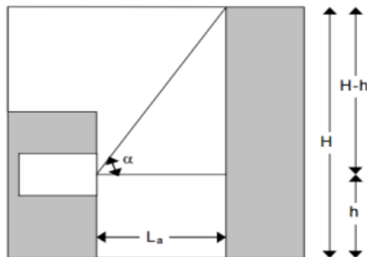
Figura 1 Valore del fattore finestra \varepsilon per ostruzioni poste di fronte alla finestra del locale considerato.
