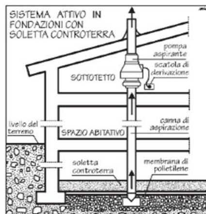
Fig.3 Sistema attivo.
