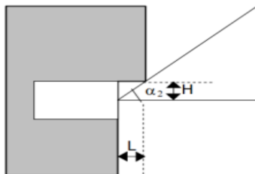
Figura 2 Valore del fattore finestra \varepsilon per ostruzioni superiori
